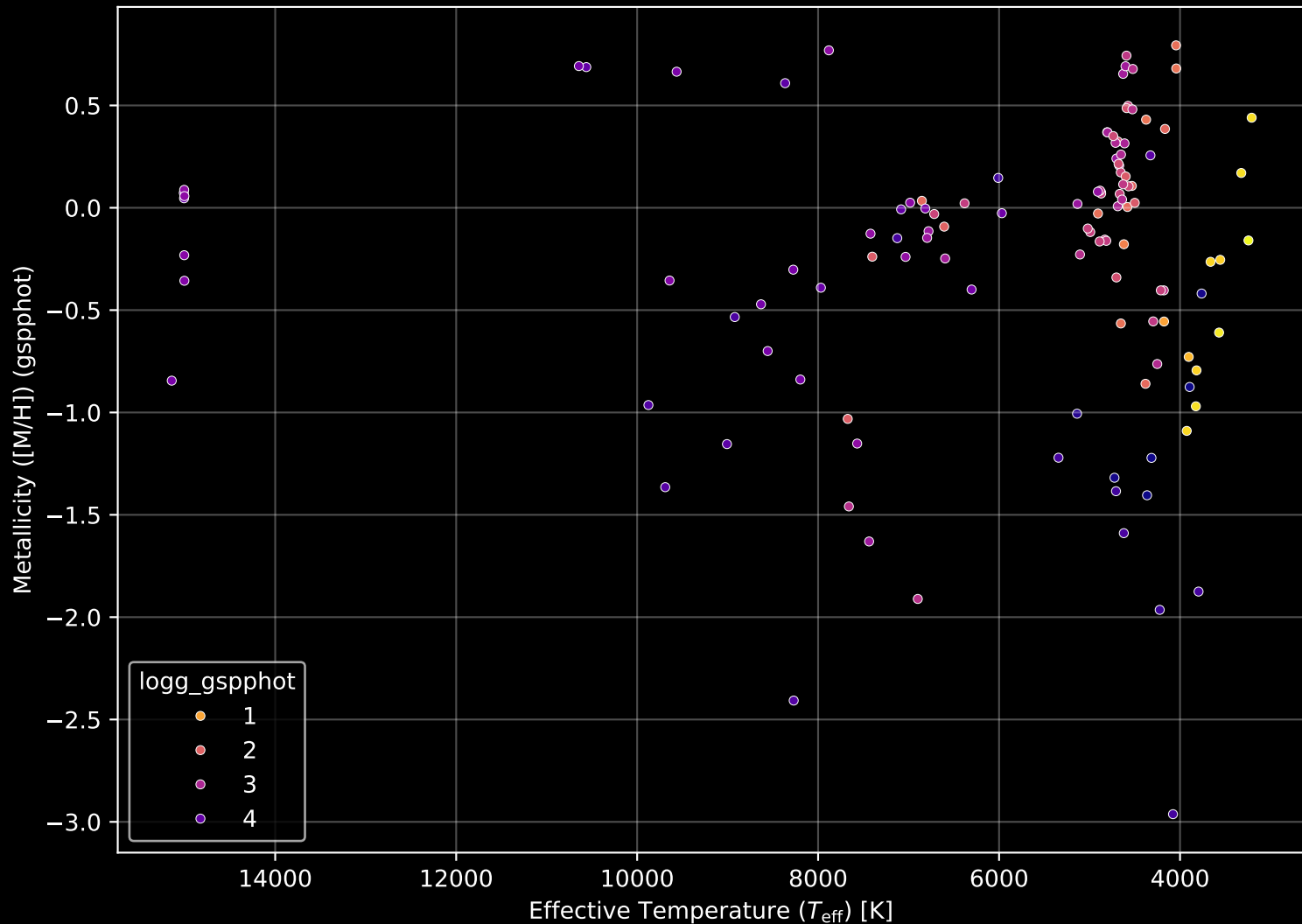
APOGEE DR17 Field: [345+00] Stellar Population Parameters (n= 120)
